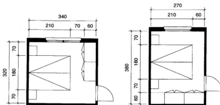
Eksempel på parsengsrom. Mål 1:100
