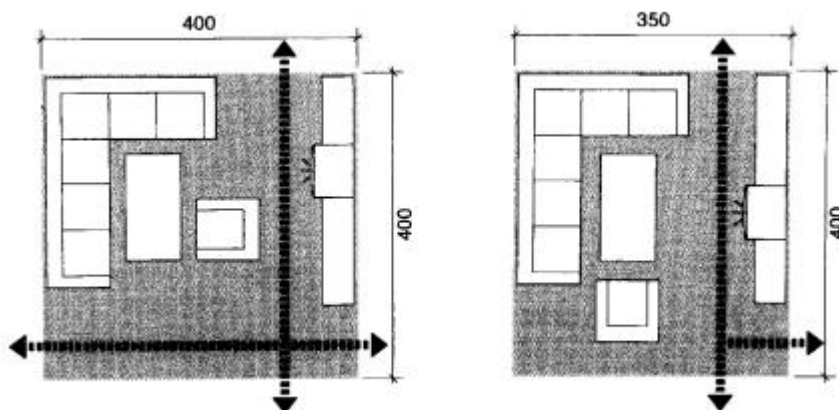
Nødvendig plass til sofagruppe, reol og passasje. Mål 1:100
