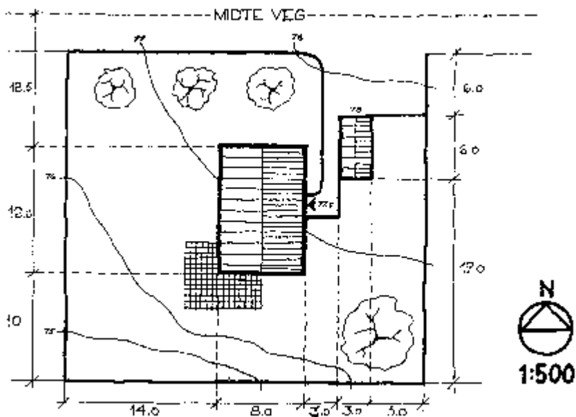
Eksempel på situasjonsplan
