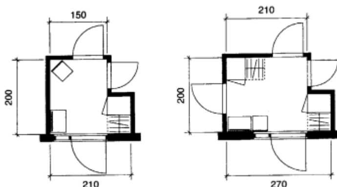
Eksempel på entre til henholdsvis 2- og 4-roms bolig. Mål 1:100
